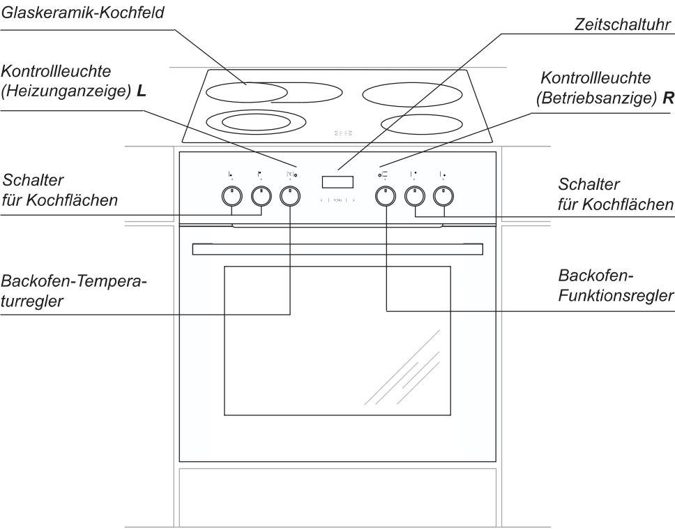
Glaskeramik-Kochfeld
