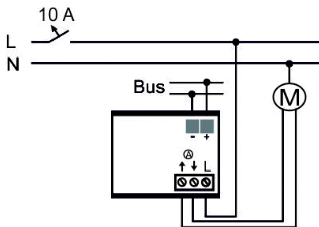
Anschlussbild
