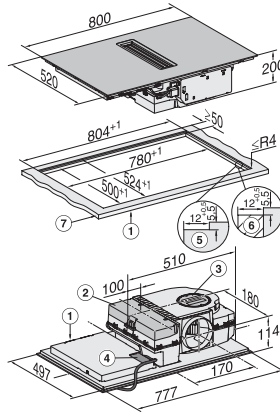
KMDA7272FL, KMDA7473FL – flächenbündig – Skizze
