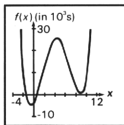
Graph von f(x)
