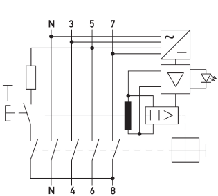
Anschlusschema
