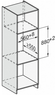
ESW7x20, Skizze
