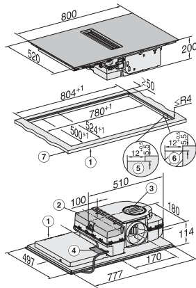
KMDA7272-1FL, KMDA7473-1FL, KMDA7272FL, KMDA7473FL – flächenbündig
