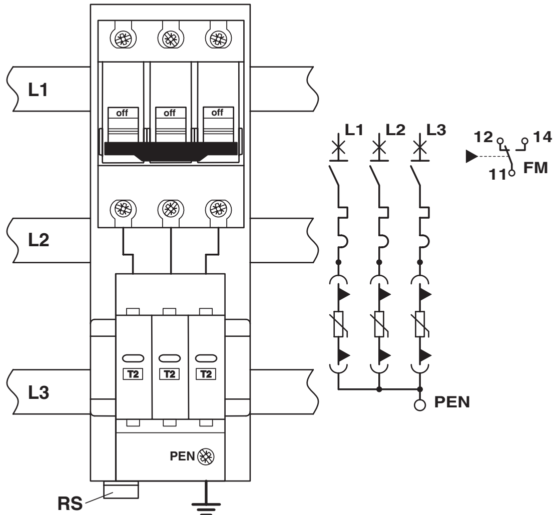
Applikationszeichnung
