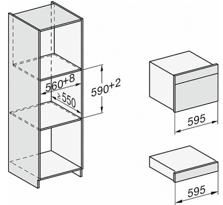
ESW7x10, Skizze
