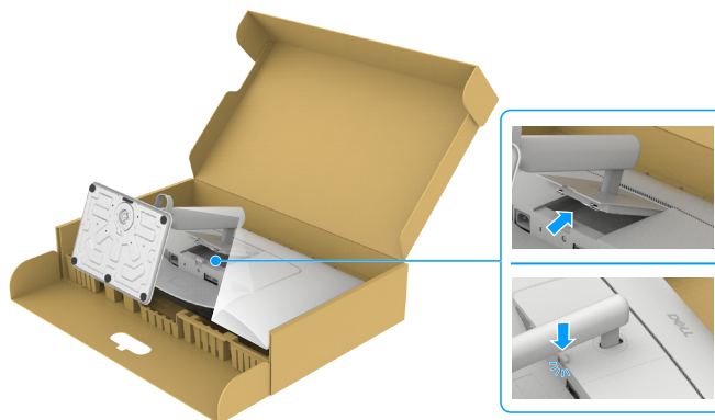
Abbildung 15. Stecken Sie die Laschen des Ständers in die Schlitzte
