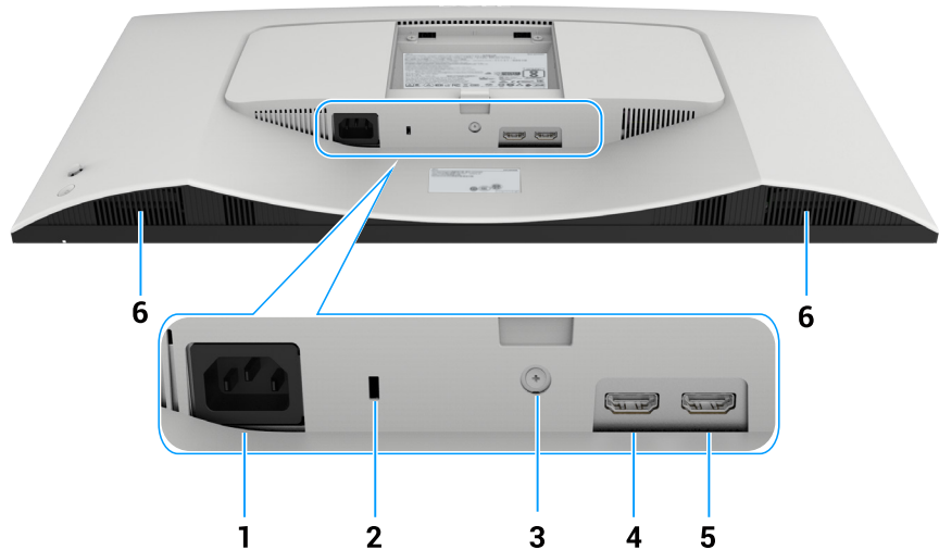
Abbildung 6. Ansicht von unten
