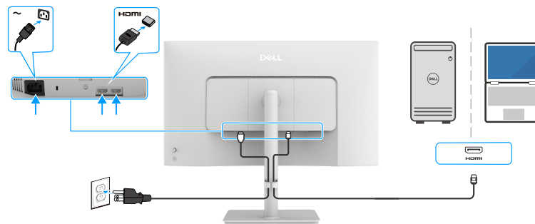
Abbildung 21. Anschließen des HDMI-Kabels
