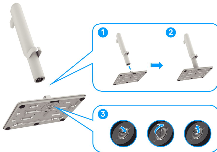
Abbildung 12. Montieren des Monitorständers
