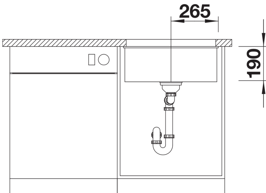
Frontansicht
