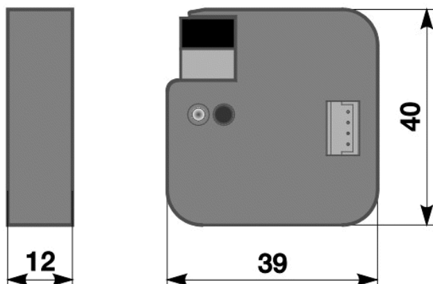
Maßbild
