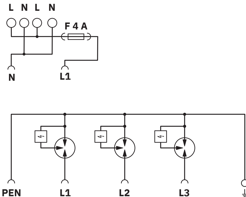
Schaltplan
