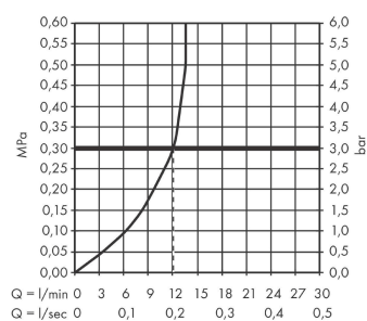
Durchflussdiagramm
