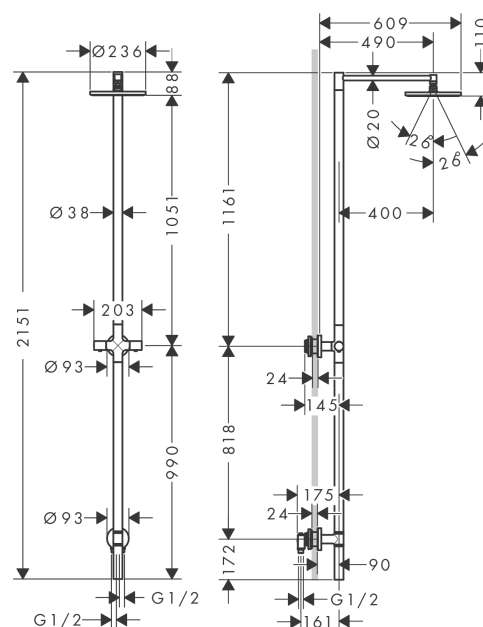
Maßzeichnung
