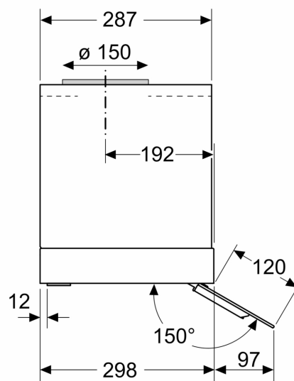
Maße in mm Seitenansicht
