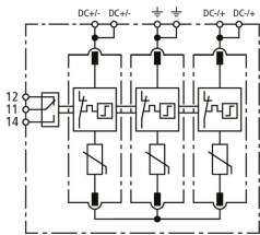
Prinzipialschaltbild DG MP YPV 1500 FM
