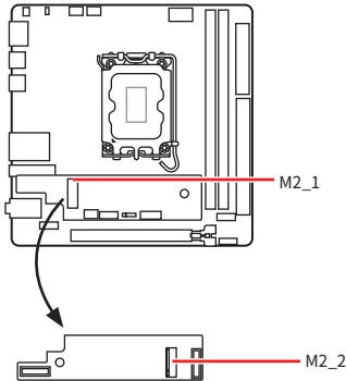
Draufsicht auf die Motherboard
