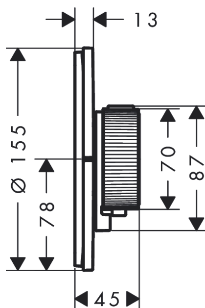
Maßzeichnung
