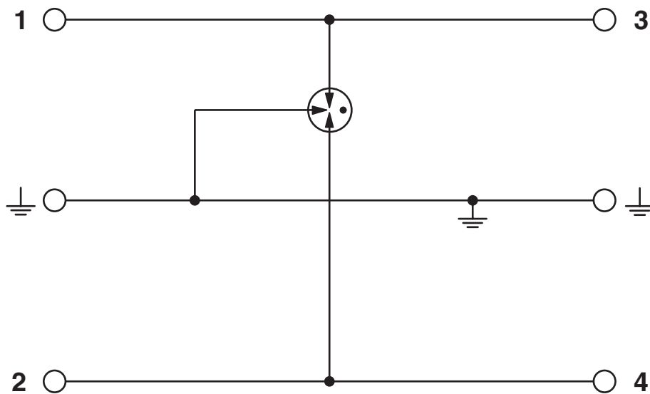
Schaltplan
