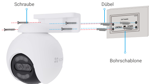
Abb. 2 Wandmontage
