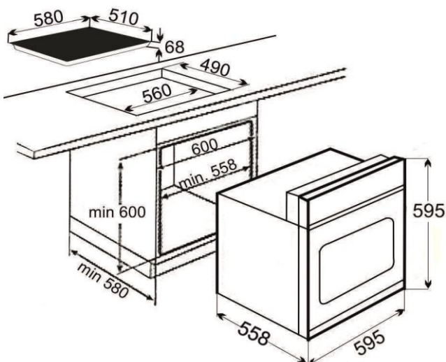
Einbauskizze
