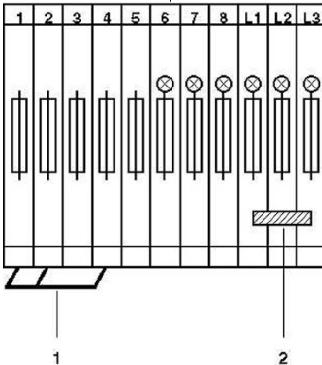
Schaltplan
