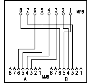
T-Adapter Cat.5 ISDN,TR / ISDN,TR 4-5, 3-6/4-5, 3-6
