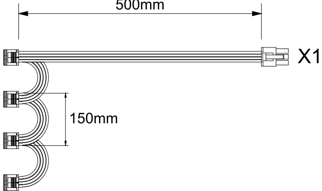
RGB SYNC 500mm
