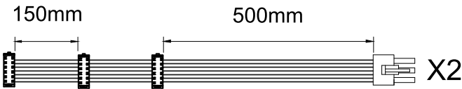
SATA CABLE
