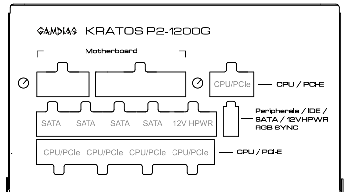
KRATOS P2-1200G
