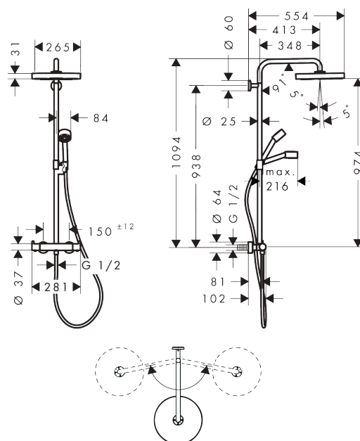
Maßzeichnung
