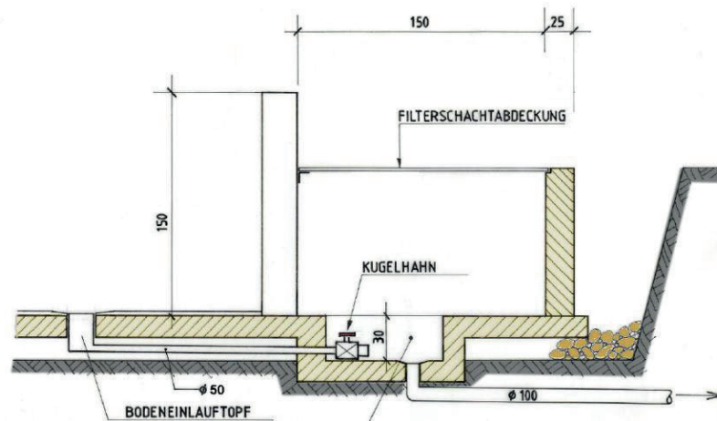
SCHNITT A-A
