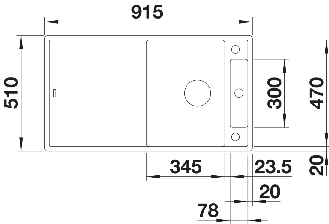
Aufsicht
