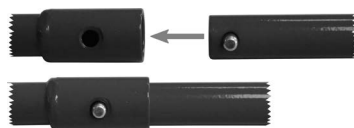
Bild 2: Pumphebel zusammenstecken
