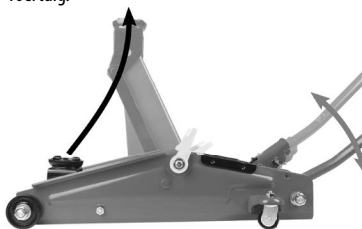
Afbeelding 3: Het voertuig optillen
