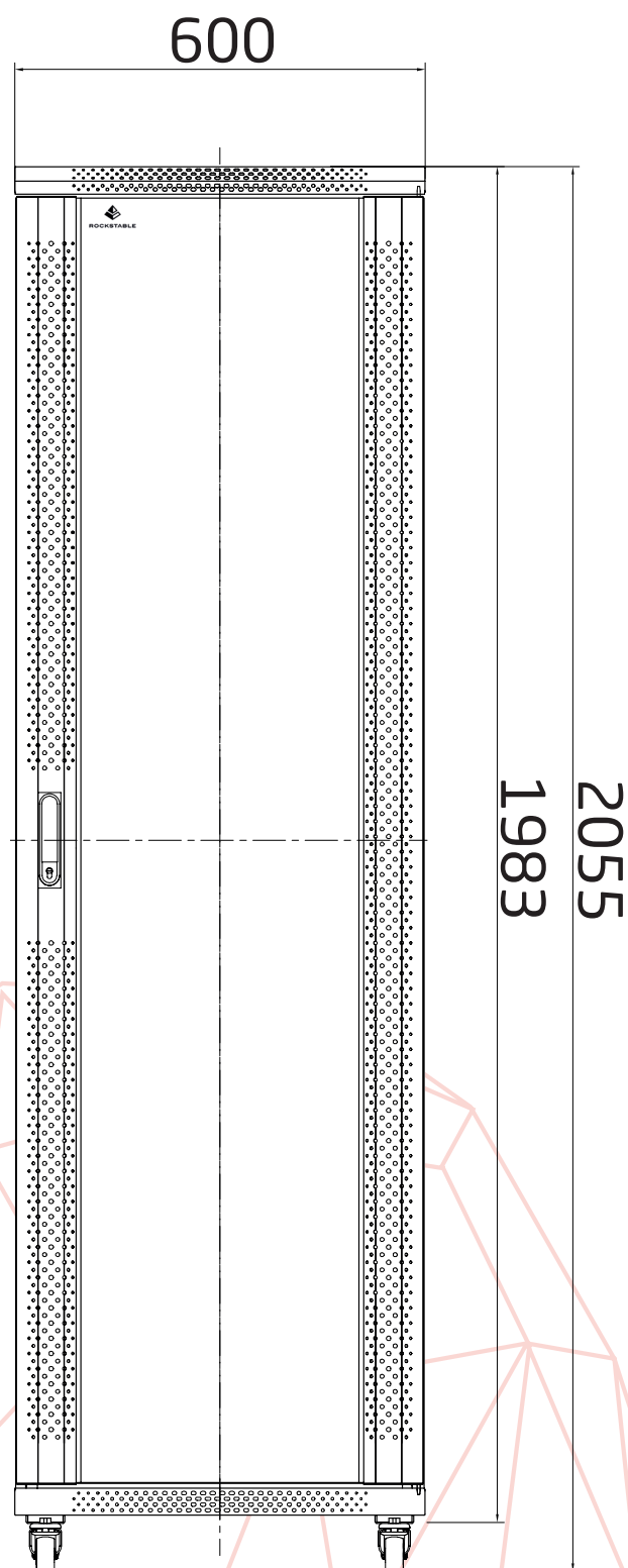
Vorderansicht
