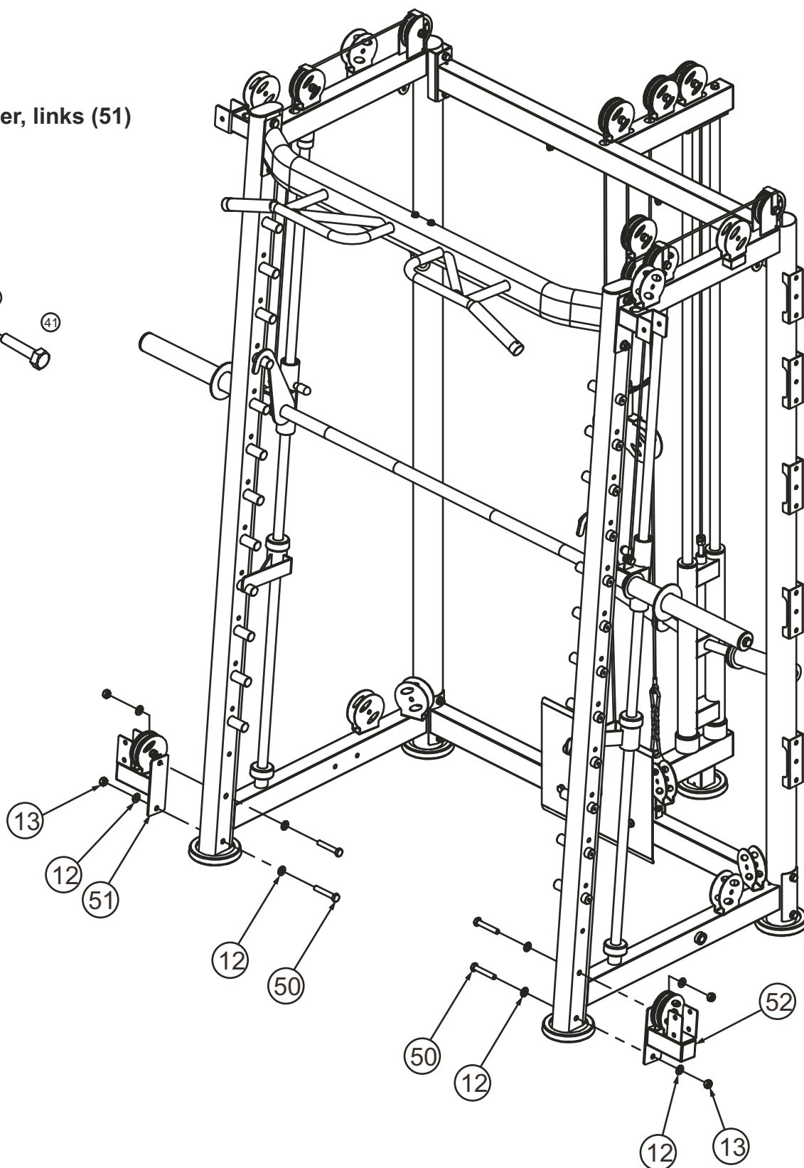
Rollenhalter, rechts (52)
