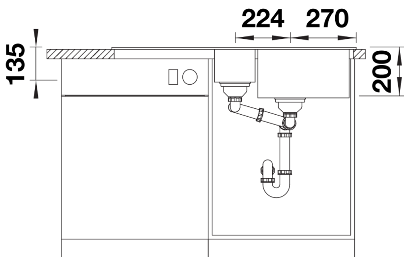
Frontansicht
