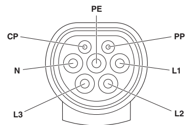
Pinbelegung Fahrzeug-Ladestecker
