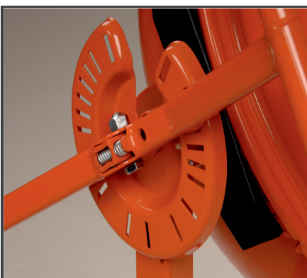
Ergonomisches und leichtgängiges Handrad mit Multirastsystem für die Mischtrommel Verstellung.
