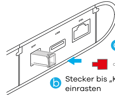
Digitalisierungsbox mit gestecktem SFP
