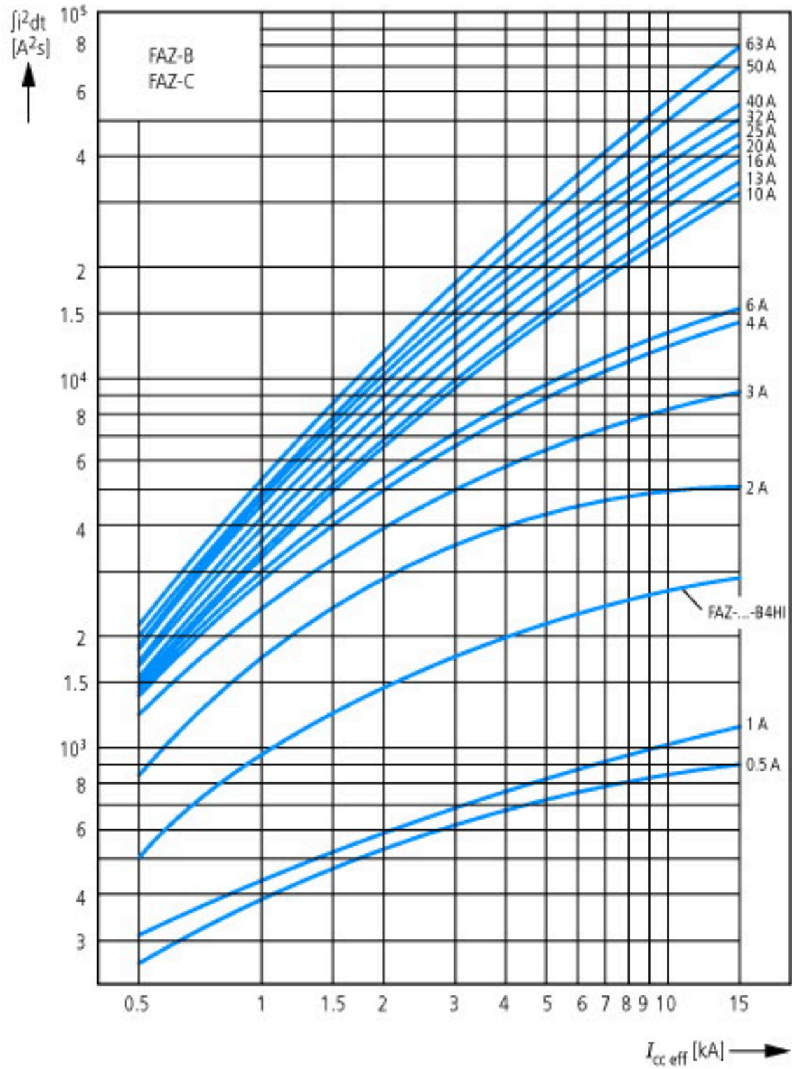
Durchlassenergie I^2t Ermittlung nach IEC/EN 60898
