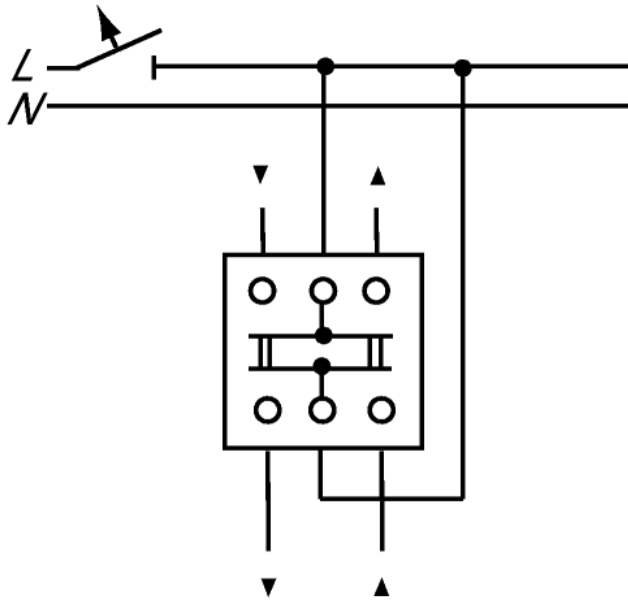
Jalousieschalter-taster, 1 P+N+PE, Drehgriff oder Schlüssel 2713-... und 2733-...
