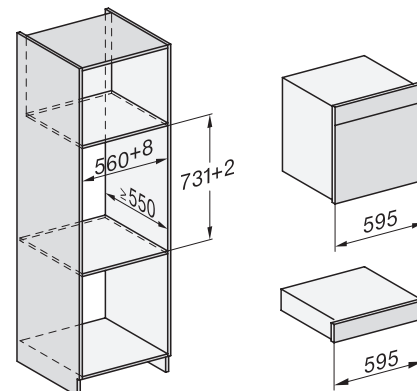
Einbau_DGC_XXL_ESW7x10_EVS7010, Skizze
