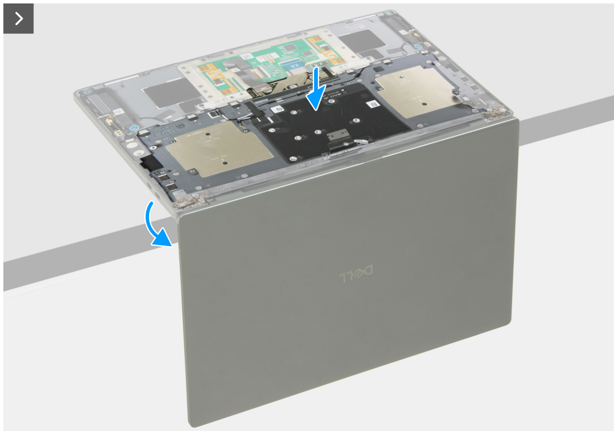
Abbildung 75. Einbauen der Tastatur
