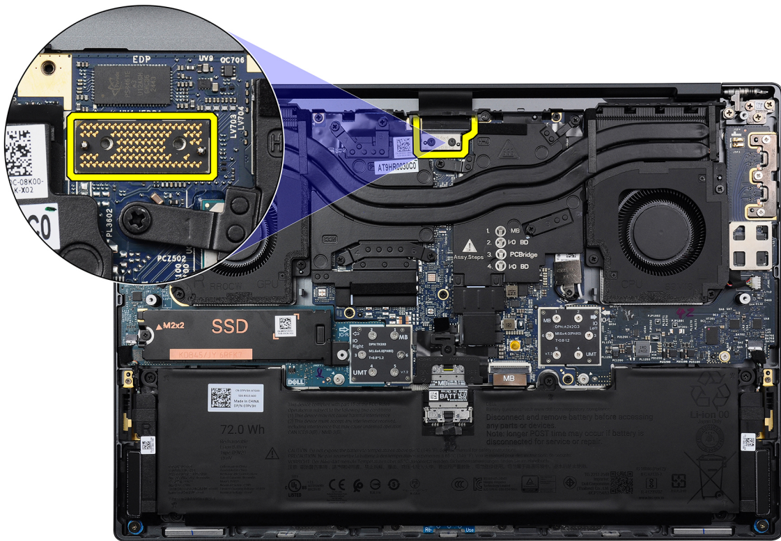
Abbildung 40. Kabelzwischenplatine der Bildschirmbaugruppe
