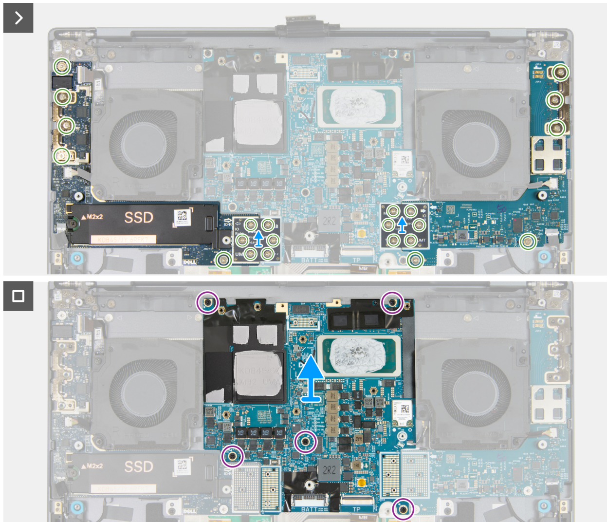
Abbildung 51. Entfernen der Hauptplatine (integrierte Grafikkarte)
