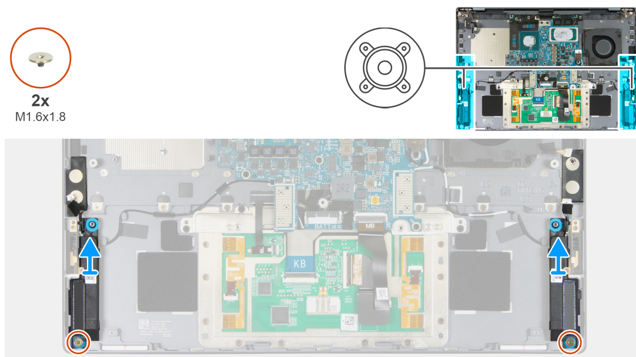
Abbildung 69. Entfernen der Lautsprecher
