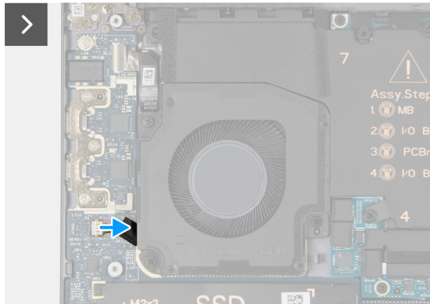
Abbildung 29. Entfernen des rechten Lüfters
