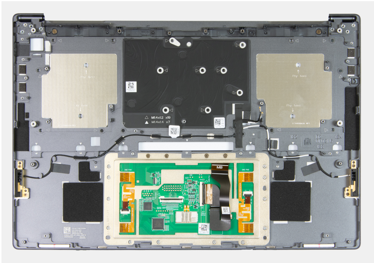
Abbildung 78. Handballenstützen- und Touchpad-Baugruppe
