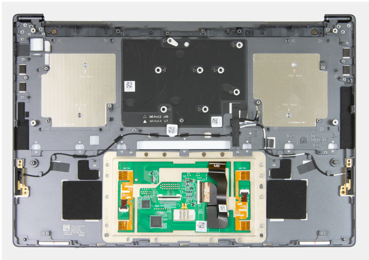
Abbildung 79. Handballenstützen- und Touchpad-Baugruppe
