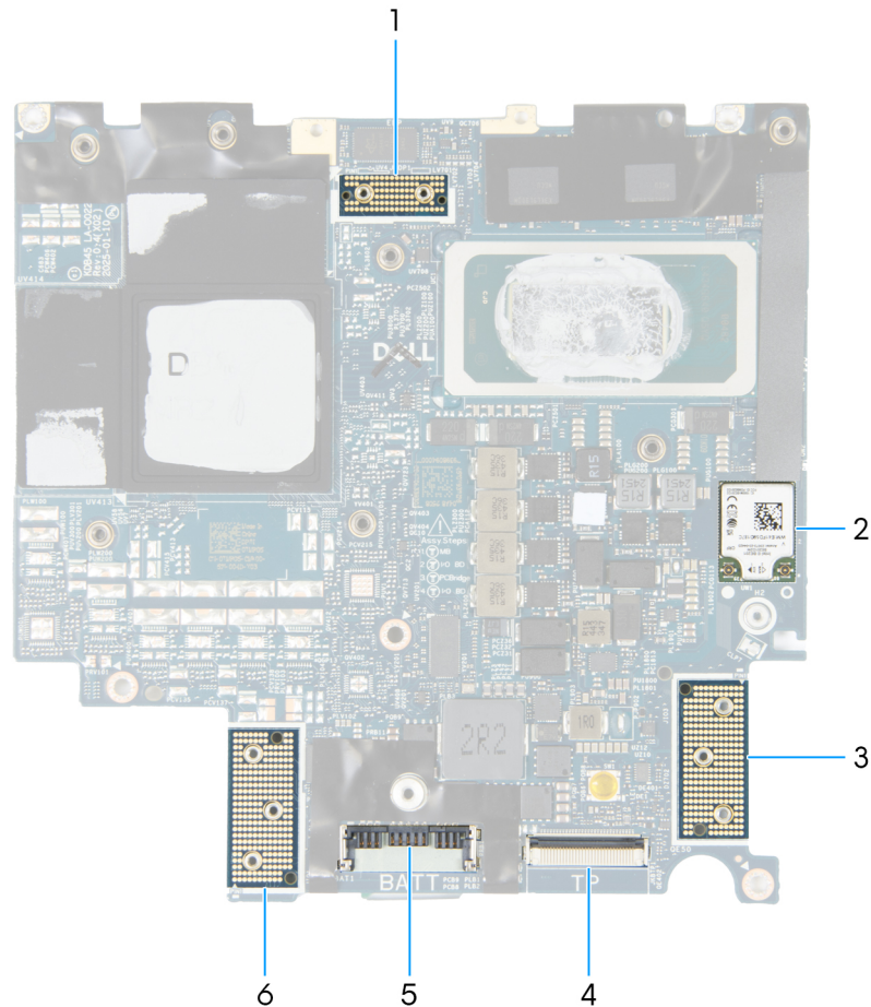
Abbildung 49. Anschlüsse auf der Hauptplatine
