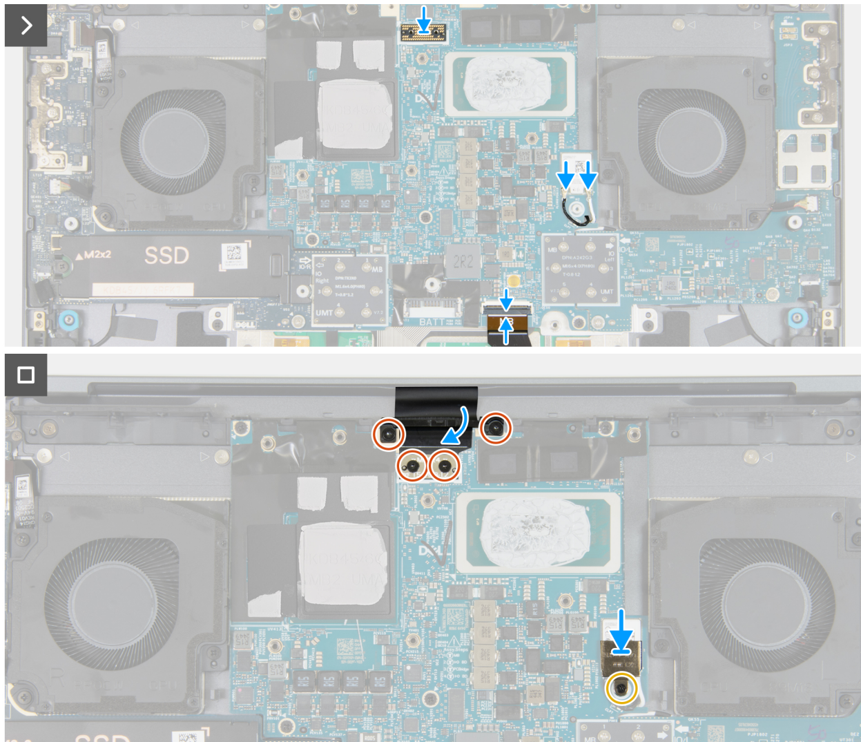
Abbildung 55. Einbauen der Hauptplatine (integrierte Grafikkarte)
