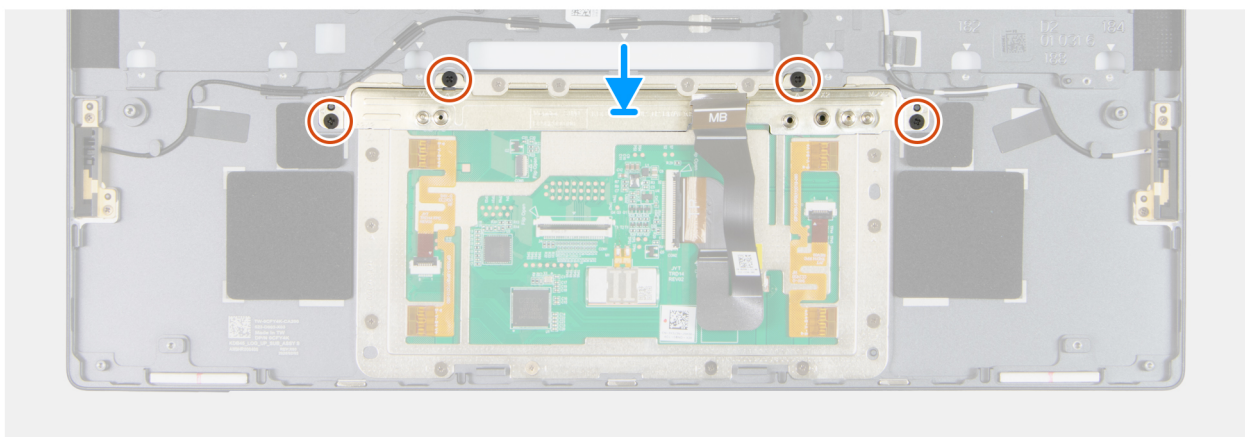
Abbildung 80. Wiedereinbau der Touchpadhalterung
