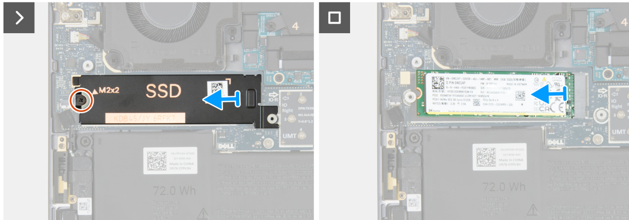
Abbildung 23. Entfernen des M.2-2280-Solid-State-Laufwerks
