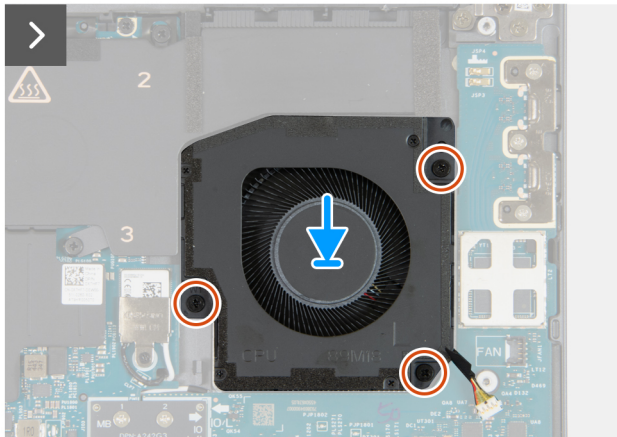
Abbildung 28. Installieren des linken Lüfters
