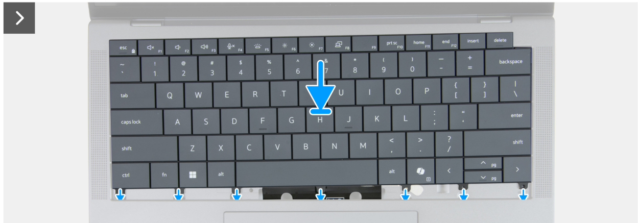
Abbildung 74. Einbauen der Tastatur
