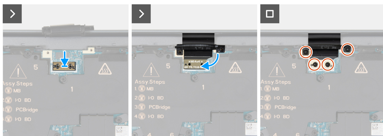
Abbildung 39. Einbauen der Bildschirmbaugruppe
