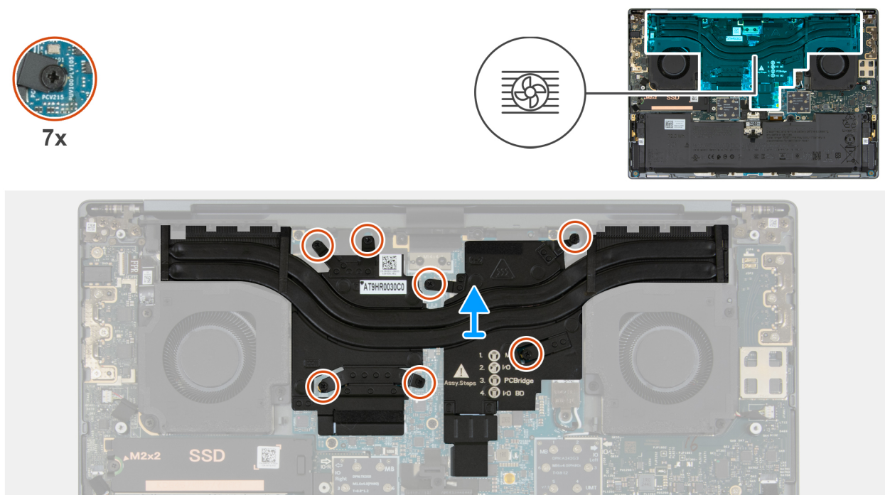
Abbildung 41. Kühlkörper entfernen
