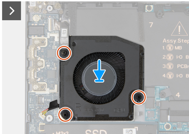
Abbildung 30. Installieren des rechten Lüfters
