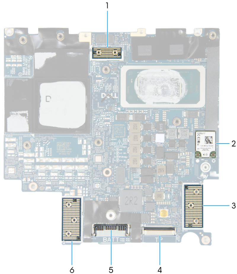
Abbildung 53. Anschlüsse auf der Hauptplatine
