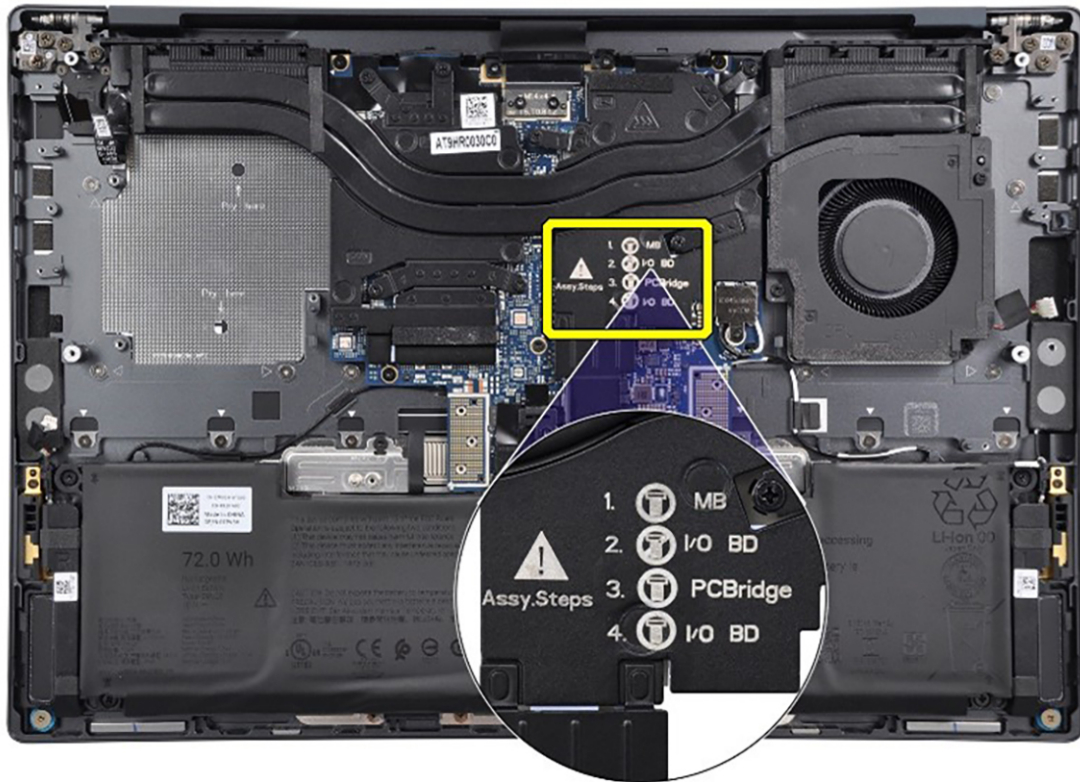
Abbildung 61. Auf dem Kühlkörper aufgedruckte Montageschritte
