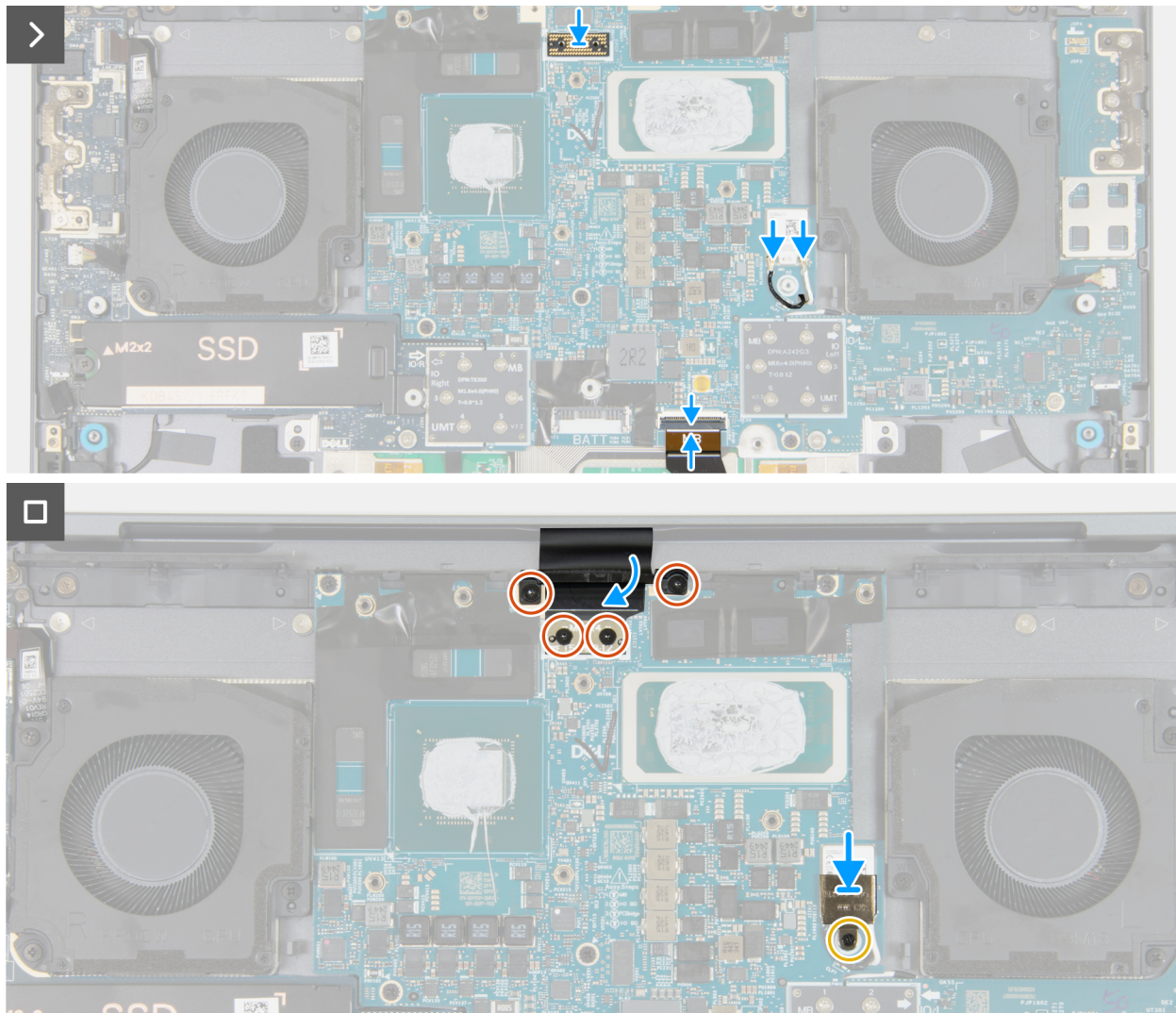
Abbildung 64. Einbauen der Hauptplatine (separate Grafikkarte)
