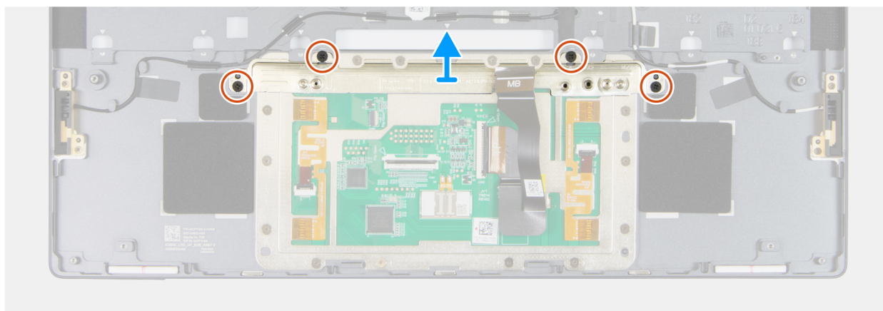
Abbildung 77. Entfernen der Touchpadhalterung
