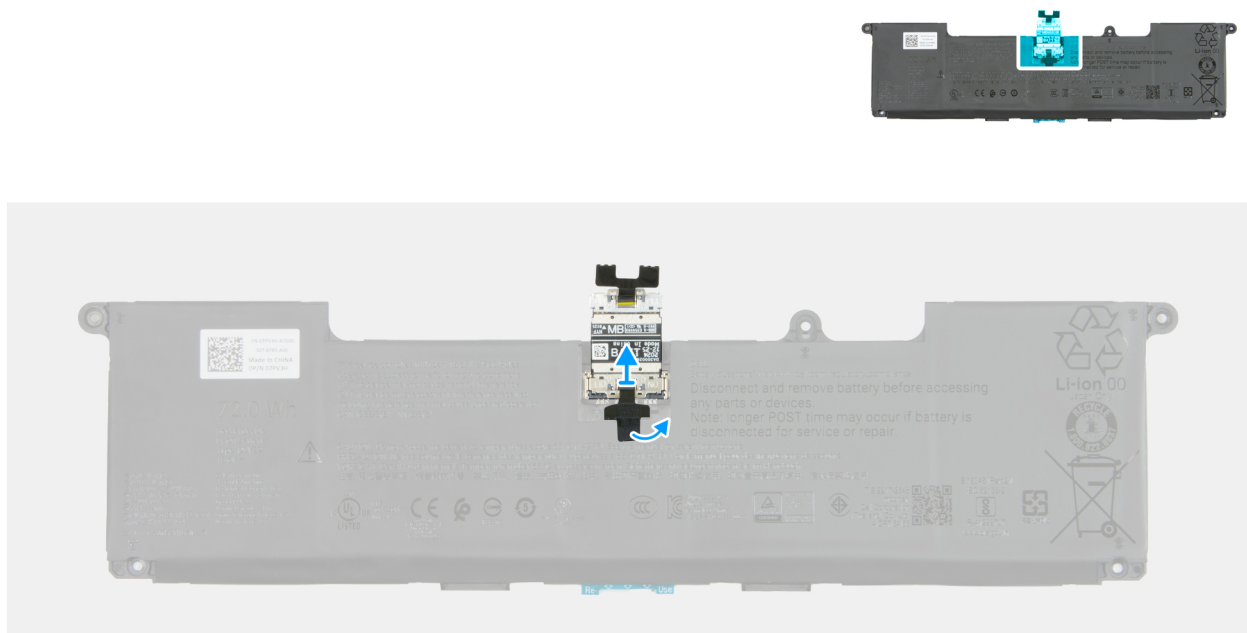
Abbildung 21. Entfernen des Akkukabels
