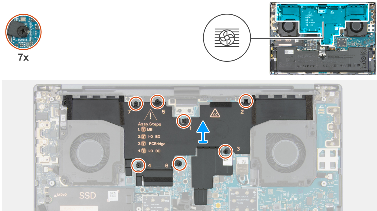
Abbildung 43. Kühlkörper entfernen
