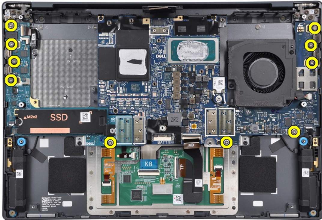
Abbildung 56. Schrauben der I/O-Platinen
