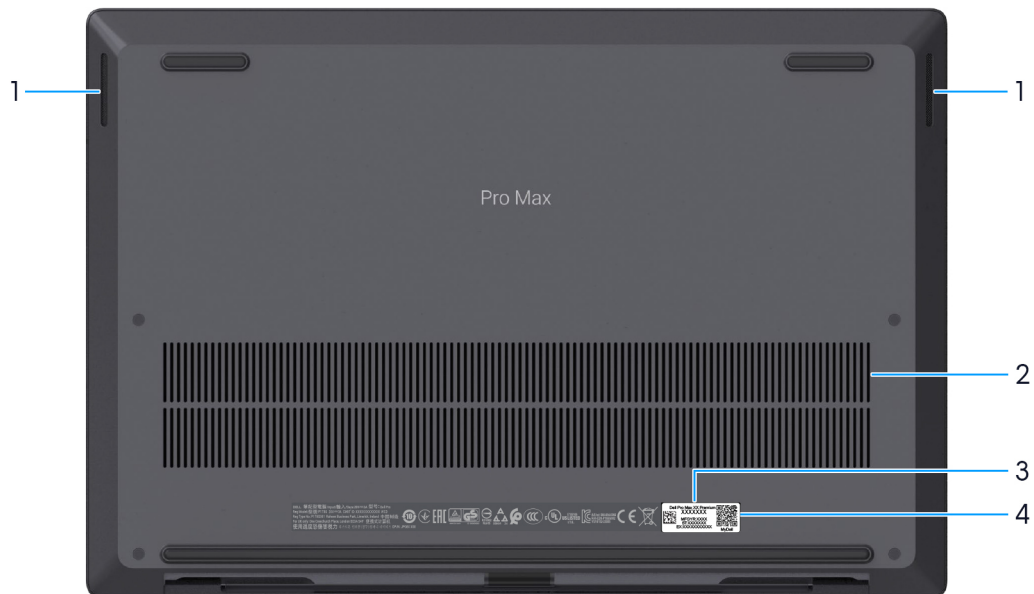
Abbildung 6. Untere Ansicht
