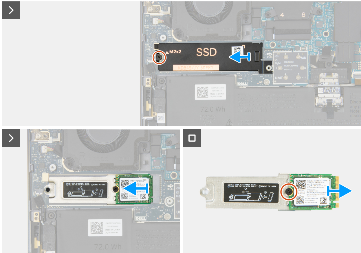
Abbildung 25. Entfernen des M.2-2230-Solid-State-Laufwerks
