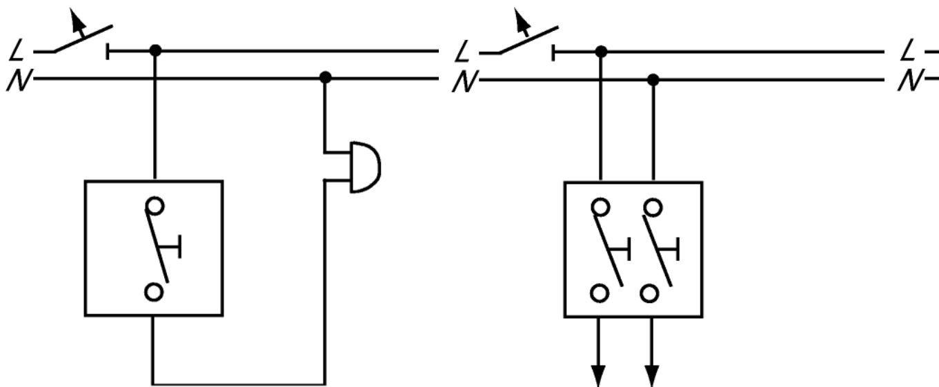
Doppeltaster, 2 Strombahnen, -205-101
