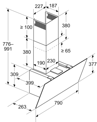
Maße in mm Gerät im Umluftbetrieb
