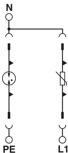
Schaltplan
