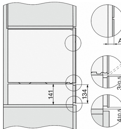
ESW7x10, EVS7010, DG7x4x, DGM7x4x Skizze
