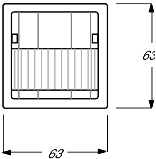
Maßbild
