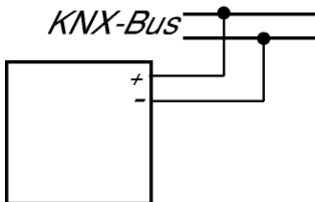
Anschlussbild
