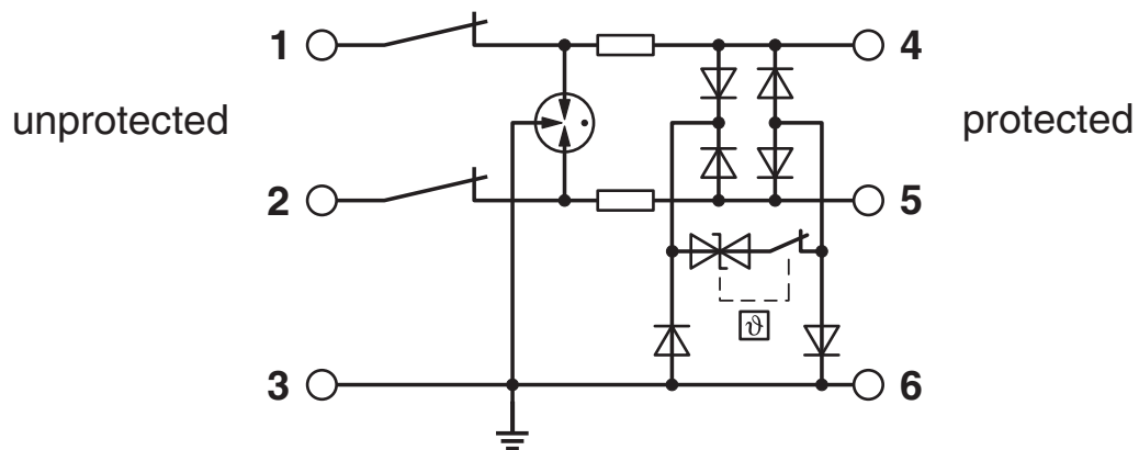
Schaltplan
