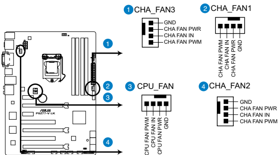
P8Z77-V LK fan connectors
