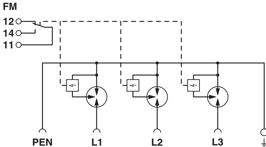
Schaltplan
