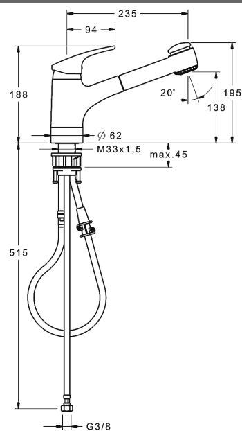
Produktzeichnung
