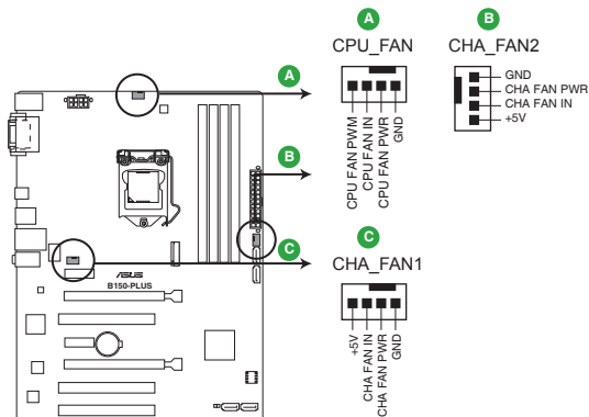
B150-PLUS Fan connectors
