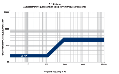
Kennlinie B NK 30 mA
