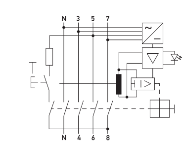
Anschlusschema
