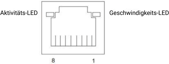
Abbildung 13. RJ45-Anschluss (Steckerseite)
