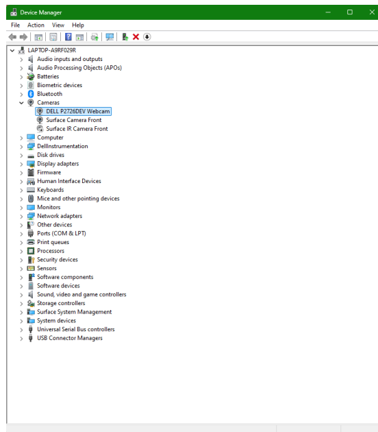
Abbildung 89. Geräte-Manager-Schnittstelle.
